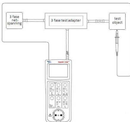
Figuur 2: Testen van 3 fase apparatuur
